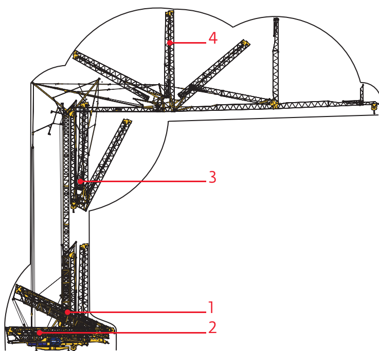
Relevage de flèche après télescopage
