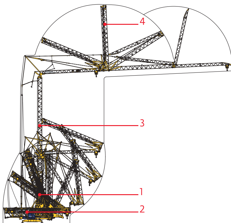
Relevage de flèche avant télescopage
